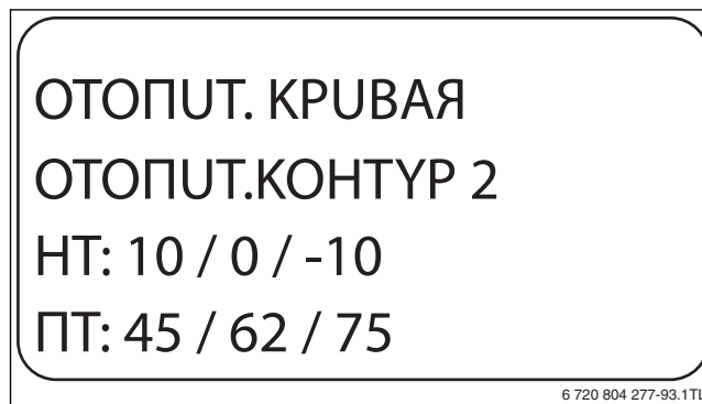
Рис. 76 Отопительная кривая
