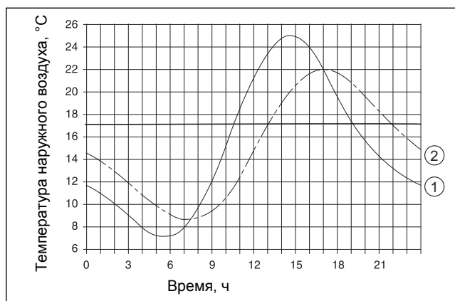
Рис. 7 Термическое запаздывание
