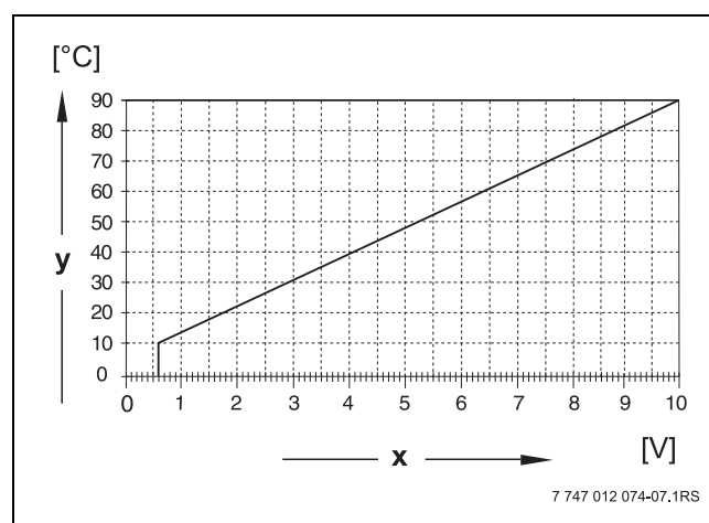
Рис. 9 U-клеммы 1 и 2
