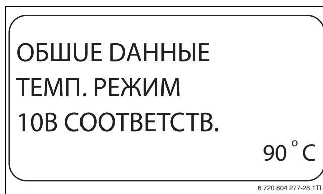
Рис. 24 Управление по температуре, вход 10 В
