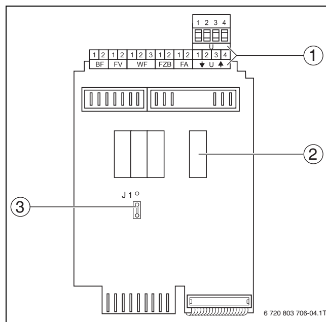
Рис. 8 ZM433 (вид сзади)
